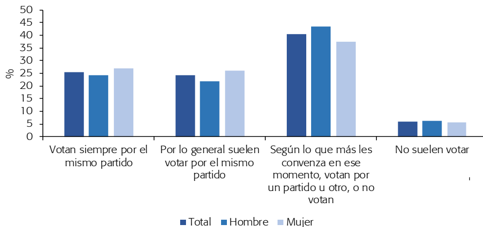
Gráfico 2 Voto crítico vs. voto fiel, por sexo (mayo 2019)
